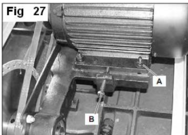
Рис. 27 Замена ремня привода врезной дисковой пилы
