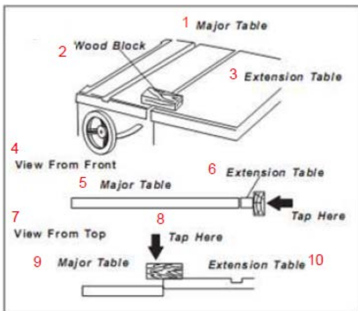
Рис. 2: 1 – главный стол, 2 – деревянная колодка, 3 – приставной стол, 4 – вид спереди, 5 – главный стол, 6 – приставной стол, 7 – вид сверху, 8 – ударить здесь, 9 – главный стол, 10 – приставной стол
